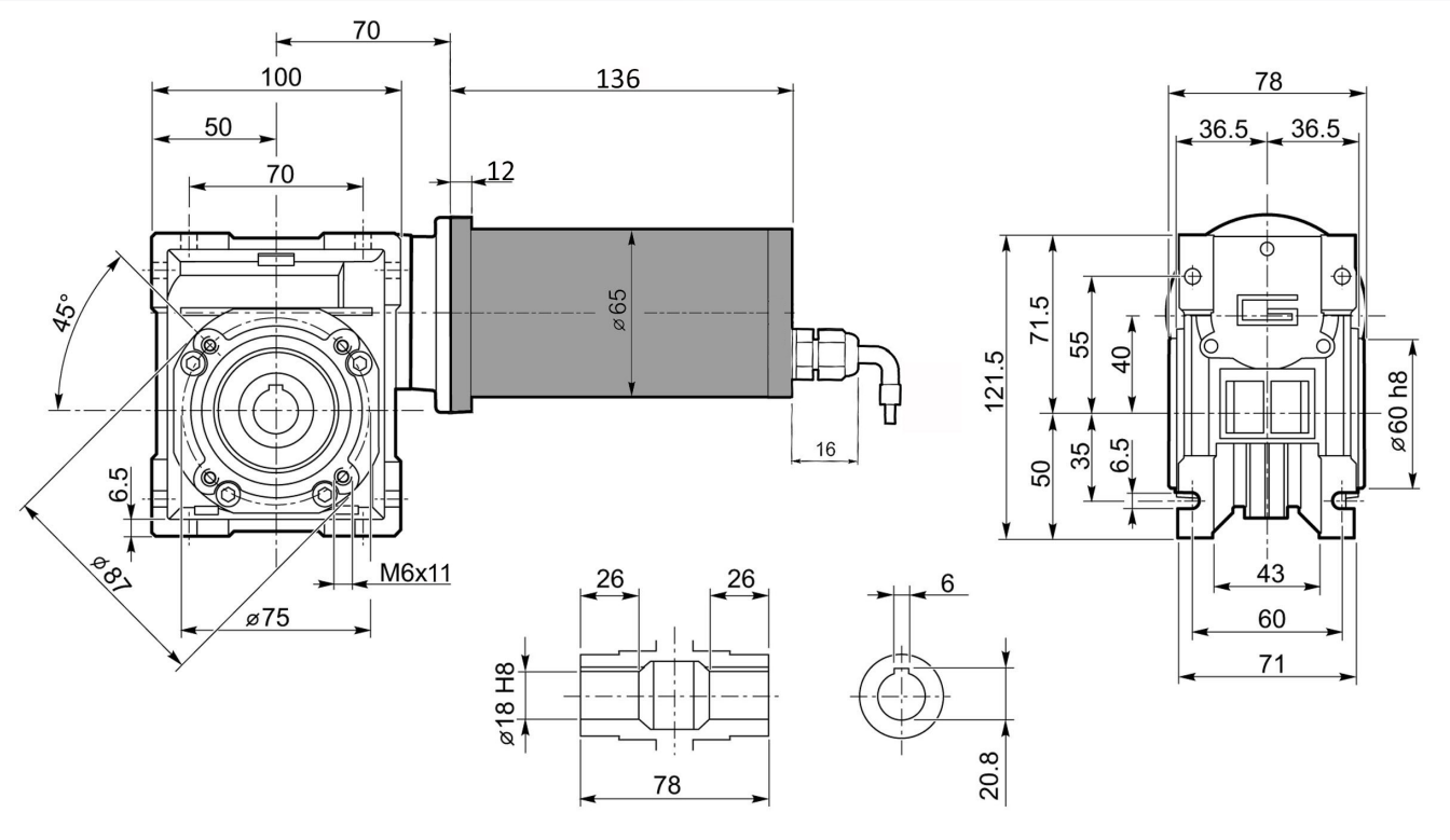
SCGS3066 mit Stirnradvorstufe
